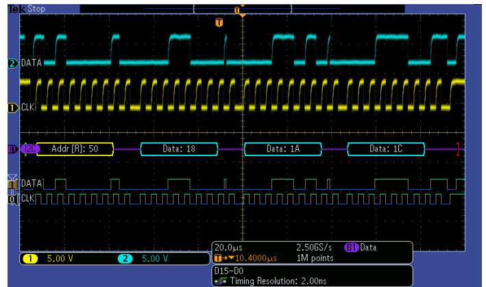
I 2 C 버스 상에서 특정 데이터 패킷에 트리거링. 노란색 파형은 클럭이며 파란색 파형은 데이터임. 버스 파형은 디코딩된 패킷 콘텐츠(Start, Address, Read/Write, Data 및 Stop)를 제공합니다.
