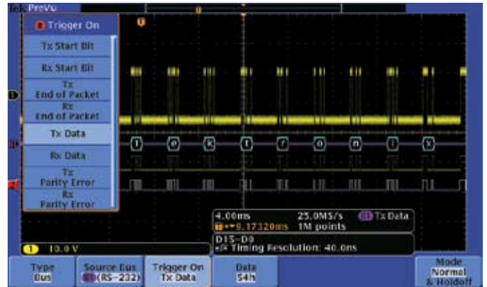
Capture – RS-232 버스 상에서 특정 전송 데이터 패킷에서 트리거링. 특정 직렬 데이터 콘텐츠의 트리거링을 포함한 트리거링을 위한 폴 세트가 제공되므로, 관심 있는 이벤트를 빠르게 캡처할 수 있습니다.
